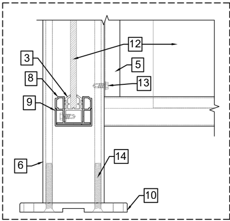
2 DÉTAIL AGRANDI
