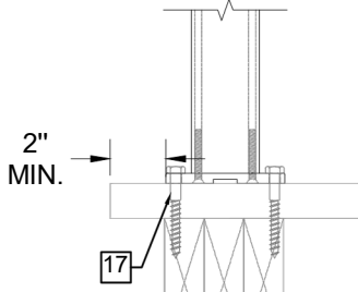
FIXATION BOIS
