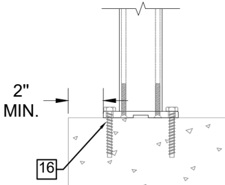
ANCRAGE BÉTON
