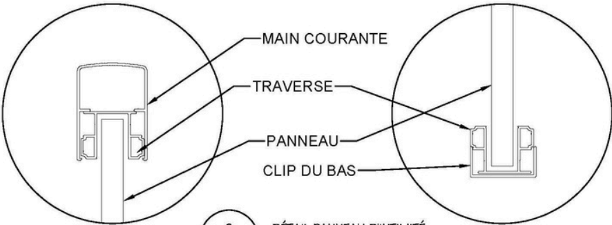
3 501 DÉTAIL PANNEAU D'INTIMITÉ
