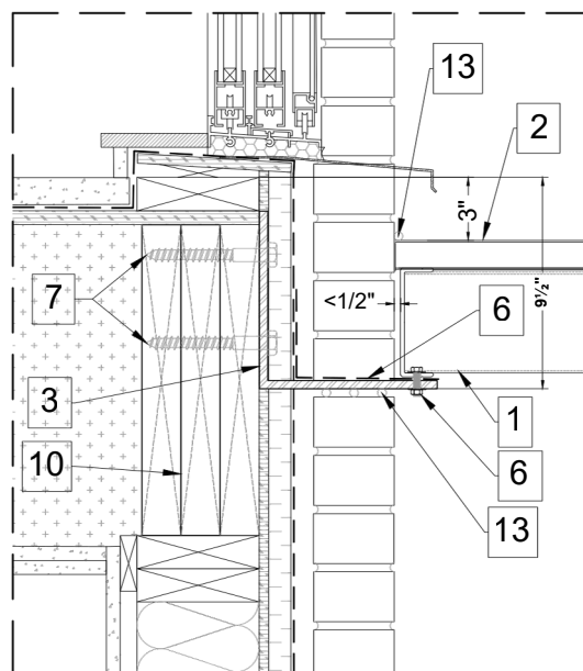
② ANCRAGE TYP. MUR AVEC BRIQUE
