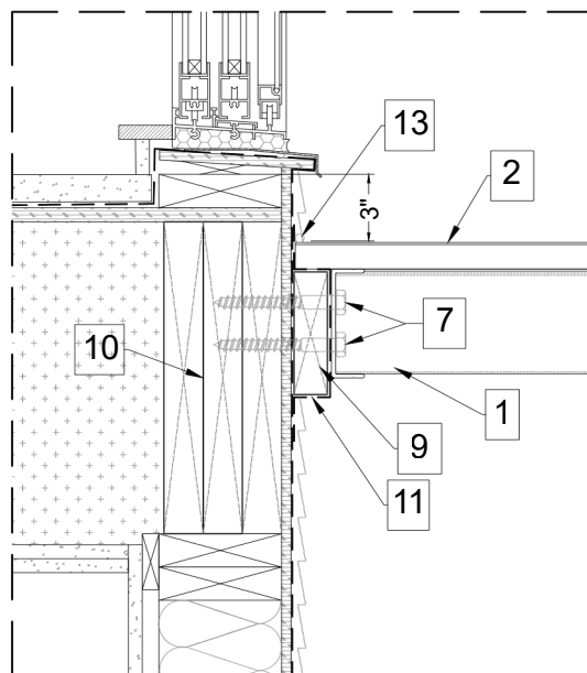
① ANCRAGE TYP. MUR AVEC REVÊTEMENT
